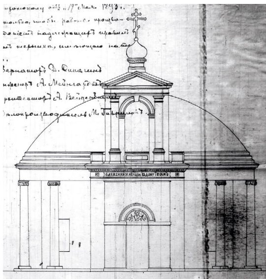
Проект реконструкции Троицкого храма
